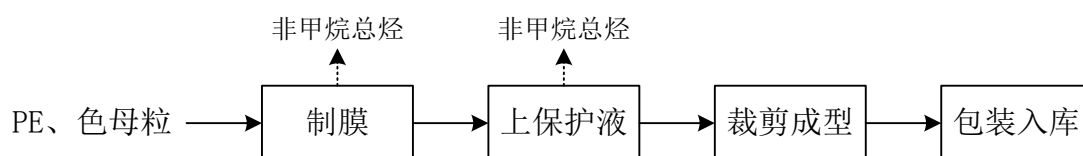
图 5-1 本项目产品的生产工艺流程及产污图
