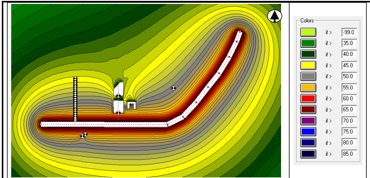
图 6-1 万兴路（亚太路-新 07 省道）段工程（K0+000~K1+450）近期昼间噪声贡献等声级线图
