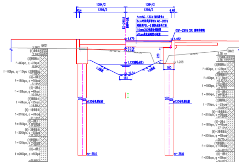
图 1-6 1 号桥立面图
